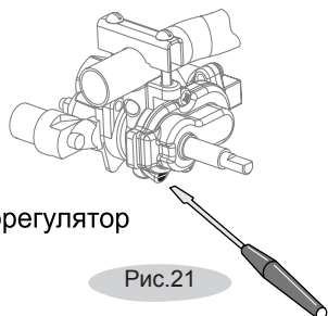
Кран без устройства контроля пламени
